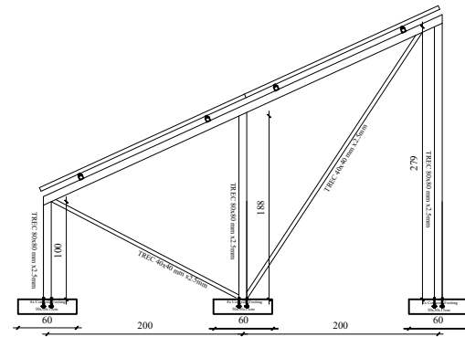
ELEVATION - 3
