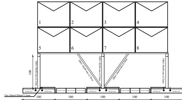
ELEVATION - 2
