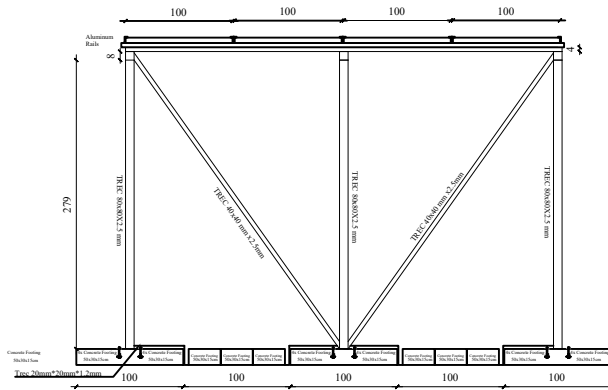
ELEVATION - 1
